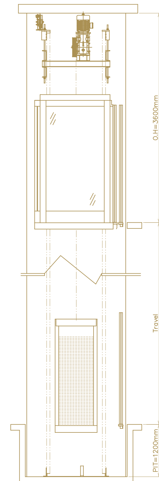
井道配置圖
