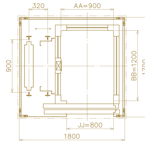
車廂配置圖
